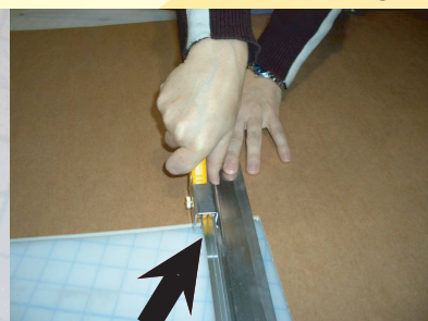
La orilla de la extrusion está donde el cuchillo corta para alineado fácil.
