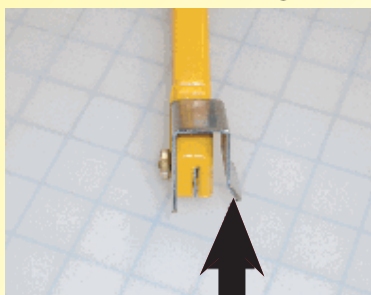
La manigueta de cuchilla sale rápido y fácilmente se monta en la extrusión guía.
